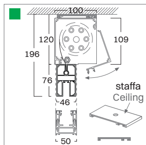
Fissaggio a soffitto con staffa Ceiling fixing
