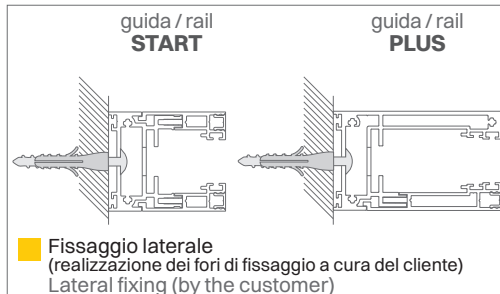
Fissaggio laterale Lateral fixing
