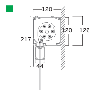
Fissaggio laterale Lateral fixing
