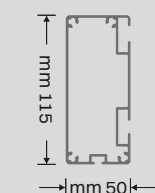
6 Trave supporto motore Motor support beam Poutre de support du moteur
